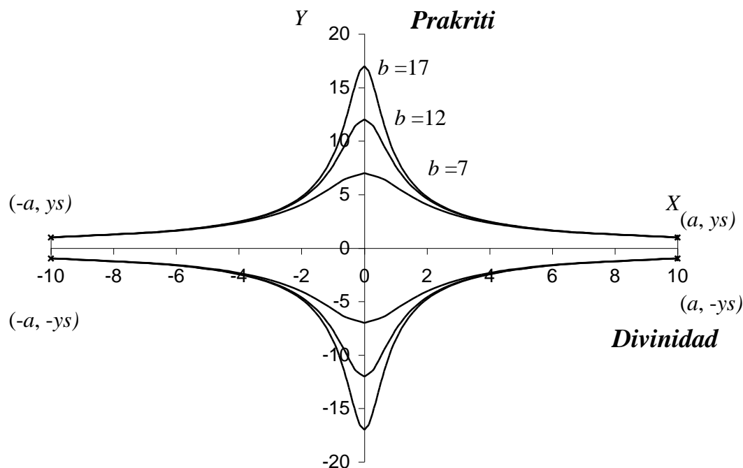
Fig. 26.2 Relatividad del Universo
