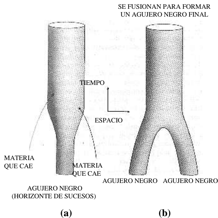
Fig. 28.2 Unión de Agujeros Negros
