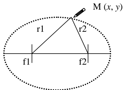
Fig. 2.3 Trazado de la Elipse
