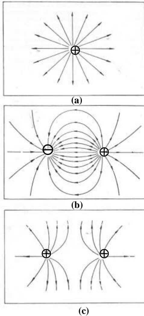
Fig. 25.4 Campo Eléctrico
