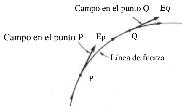
Fig 25.3 Líneas de fuerza
