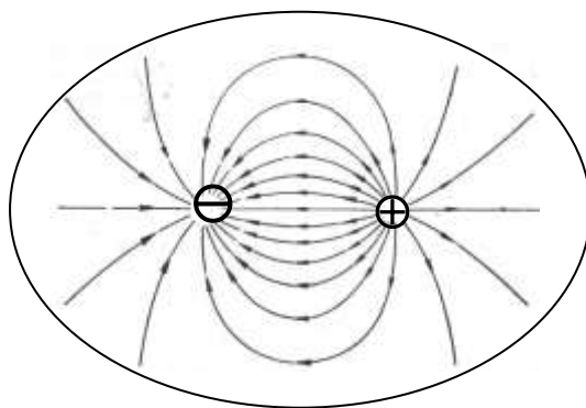
Fig 25.5 Campo del Amor o Campo del Universo
