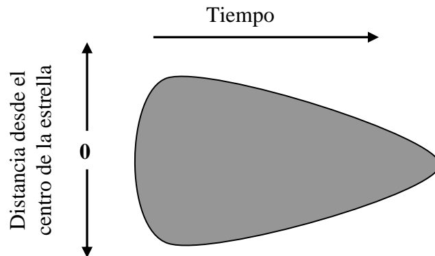
Fig. 27.3 Cono de Luz cerrándose
