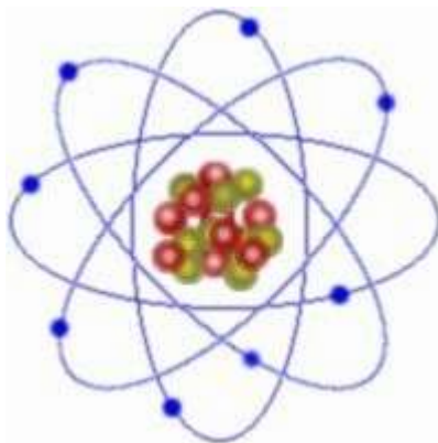
Fig. 9.1 Modelo atómico
