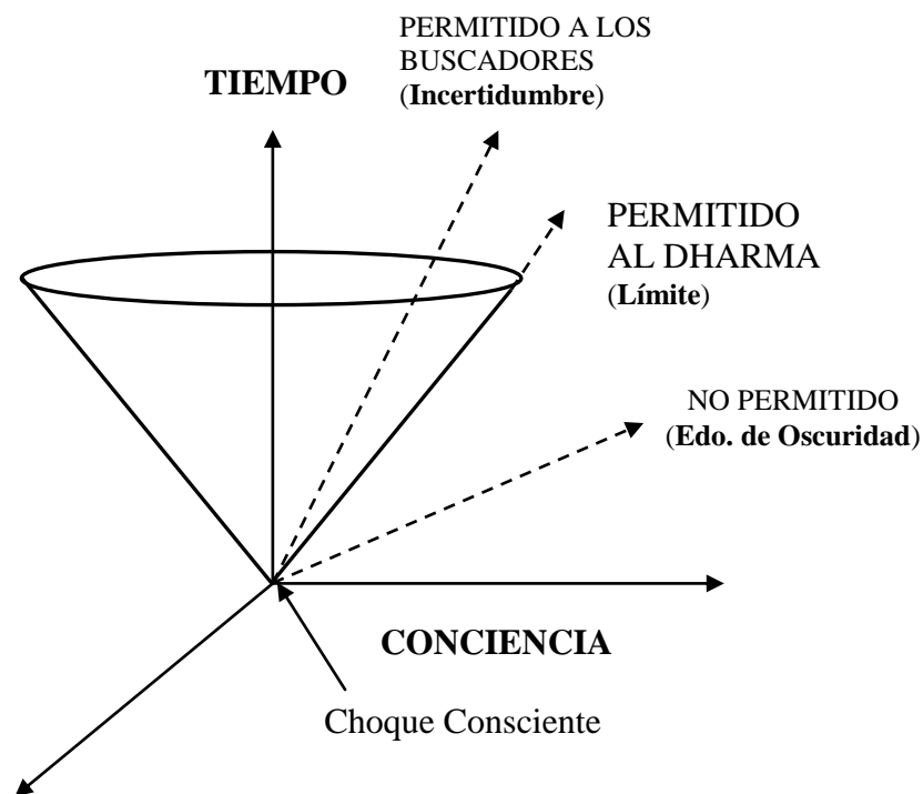
Fig. 22.3 Caminos de la conciencia y el Tiempo
