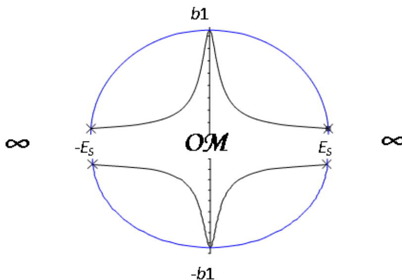
Fig. 26.3 Vía de Escape
