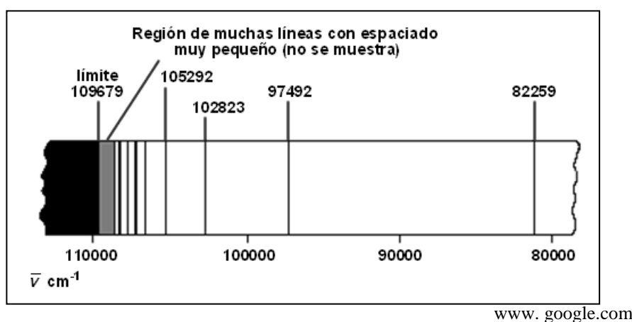
Fig. 23.1 Espectro de átomos de hidrógenos
