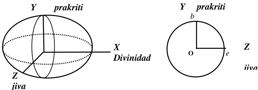
Fig. 8.1 Ciclo Nacimiento y Muerte
