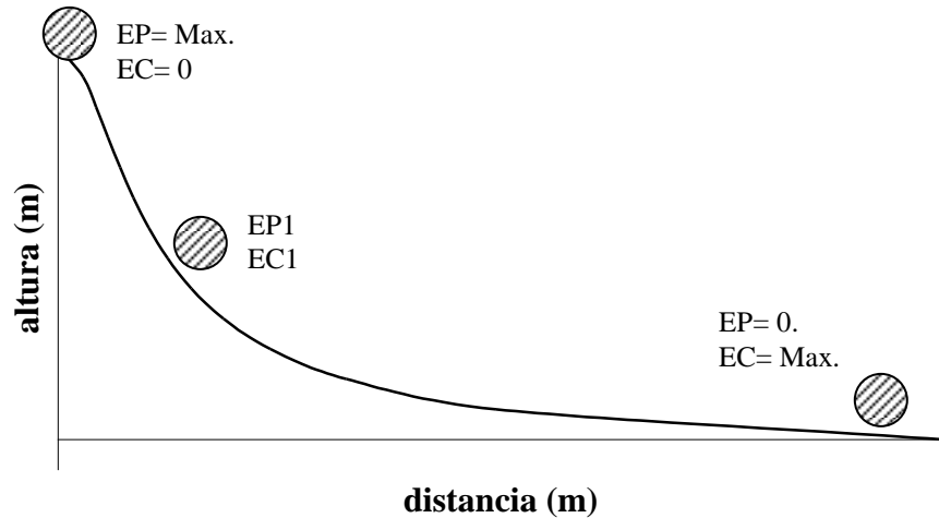
Fig. 25.6 Energía Potencial y Energía Cinética
